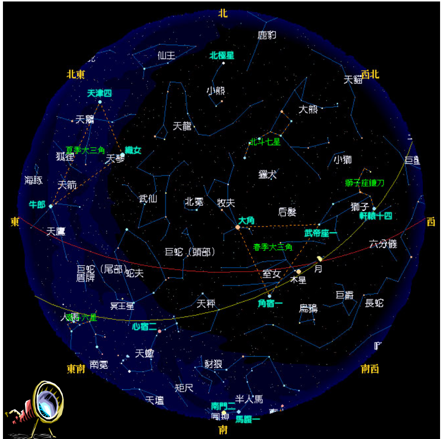
2005年6月初22:00、6月中21:00、6月底20:00的天空
